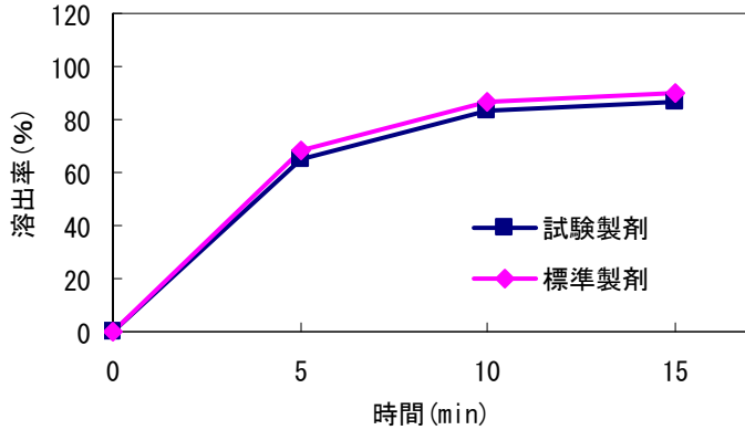
図5 パドル法(50rpm)試験液「pH7.5」における試験製剤及び標準製剤の溶出挙動
