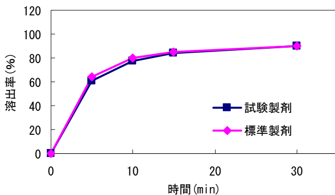
図3 パドル法(50rpm)試験液「pH5.5」における 試験製剤及び標準製剤の溶出挙動
