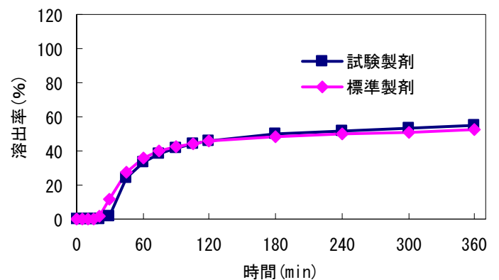
図2 パドル法(50rpm)試験液「pH6.0」における試験製剤及び標準製剤の溶出挙動
