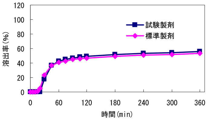
図5 パドル法(100rpm)試験液「pH6.0」における試験製剤及び標準製剤の溶出挙動
