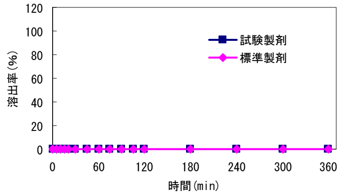
図4 パドル法(50rpm)試験液「薄いpH6.0」における試験製剤及び標準製剤の溶出挙動
